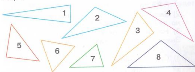
Треугольники
